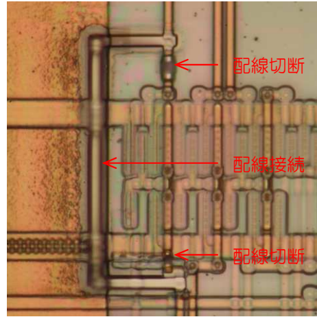
FIB加工後の金属顕微鏡像
