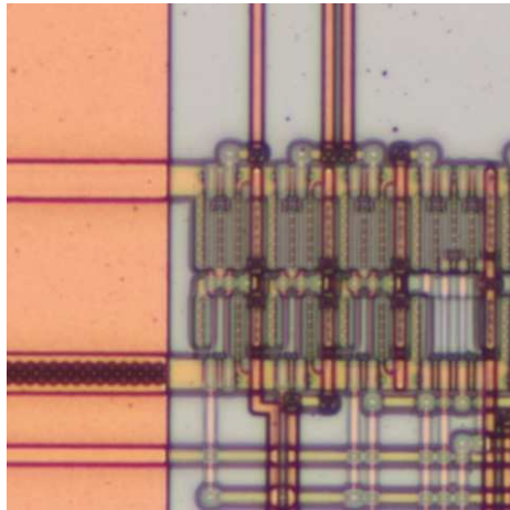
FIB加工前の金属顕微鏡像
